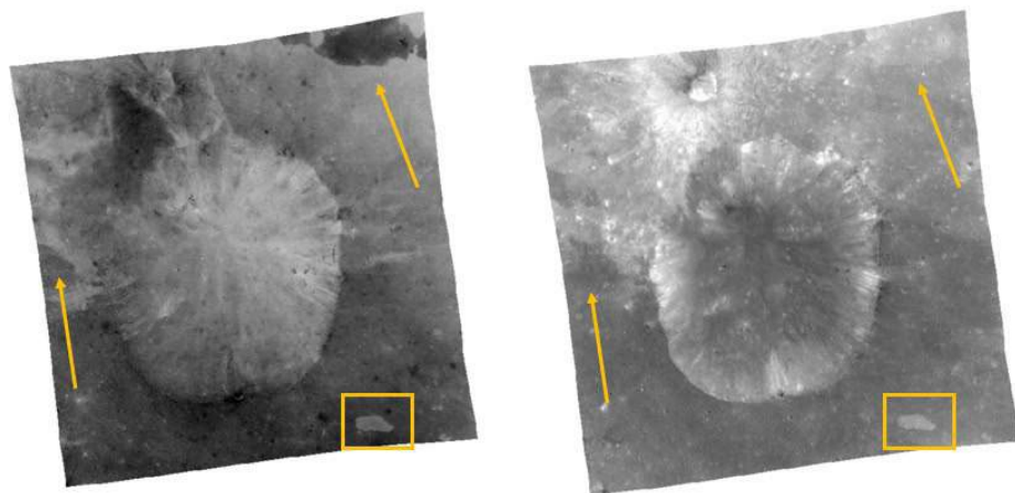
Ділянка навколо кратеру Orphea (8°S, 309°E, D=37 км). Карти розподілу колориметричних відношень C(438nm/749nm) (ліворуч) та C(749nm/917nm) (праворуч). Кілька плям, раніше класифікованих як світла мантія, показують значною мірою відмінні спектральні характеристики порівняно з традиційною спектральною поведінкою плям.
